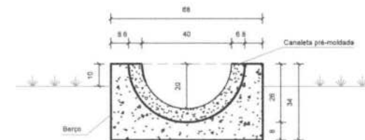
Seção transversal Sem escala
