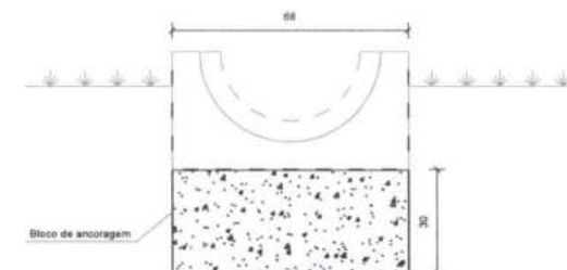
Detalhe do bloco de ancoragem Sem escala
